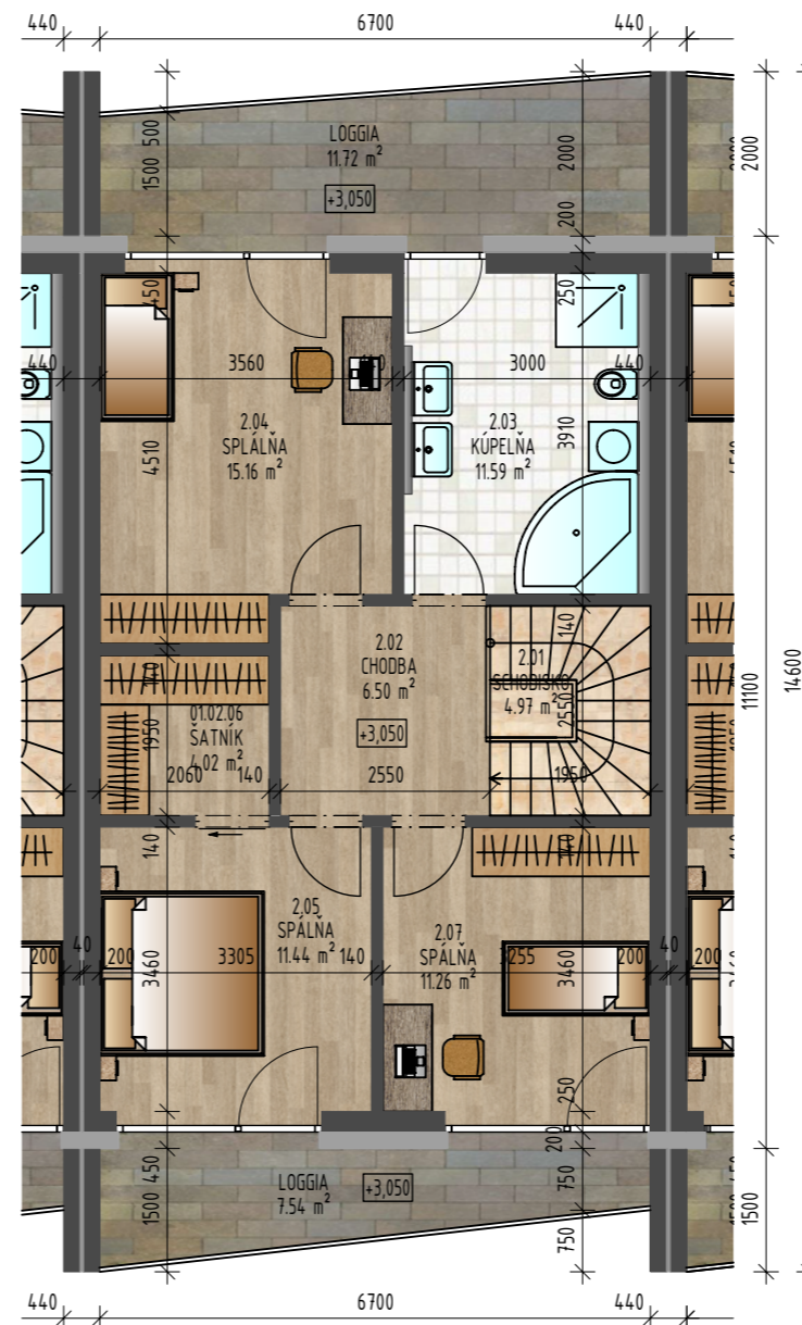
DOM I - PÔDORYS 2.NP
