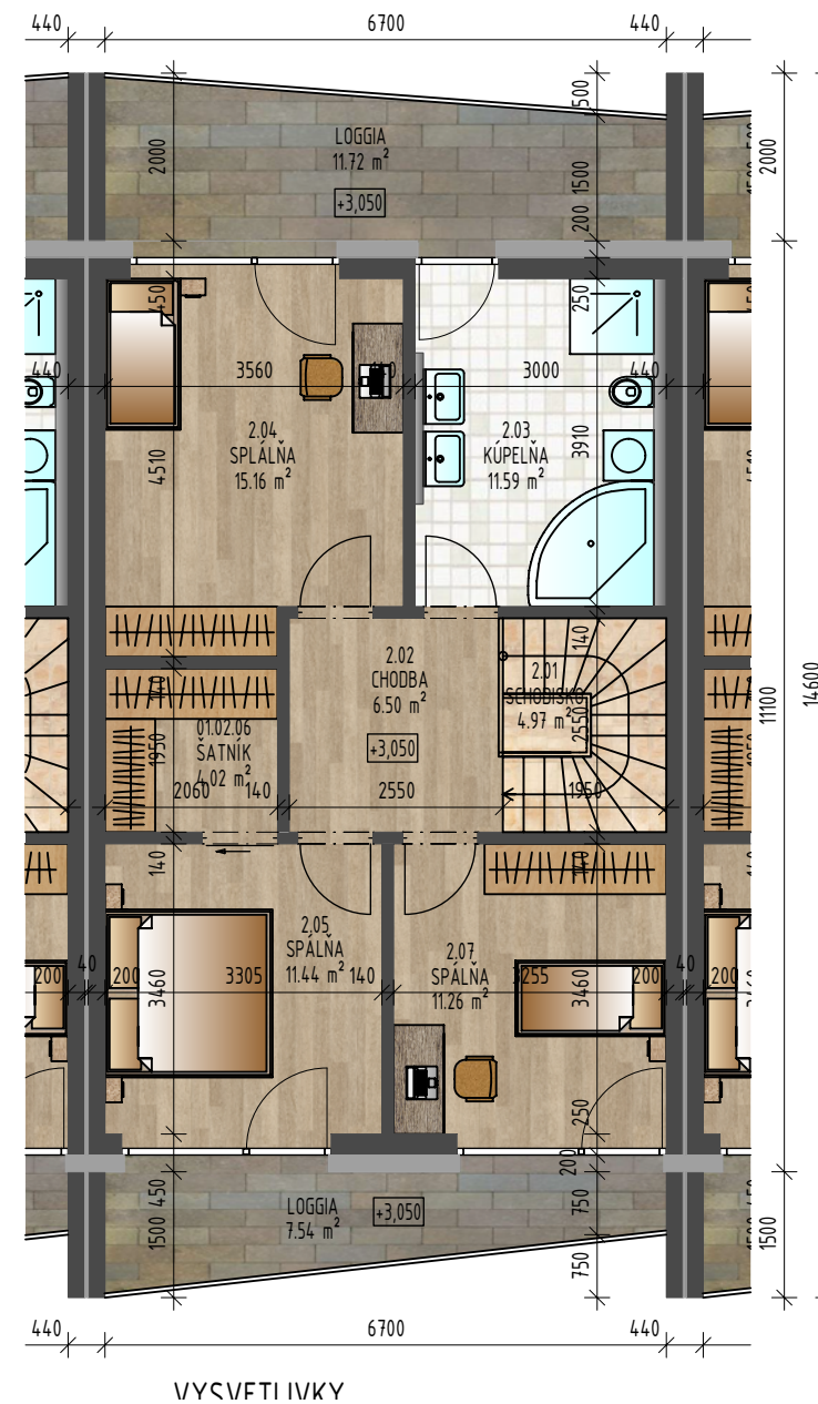
DOM D - PÔDORYS 2.NP
